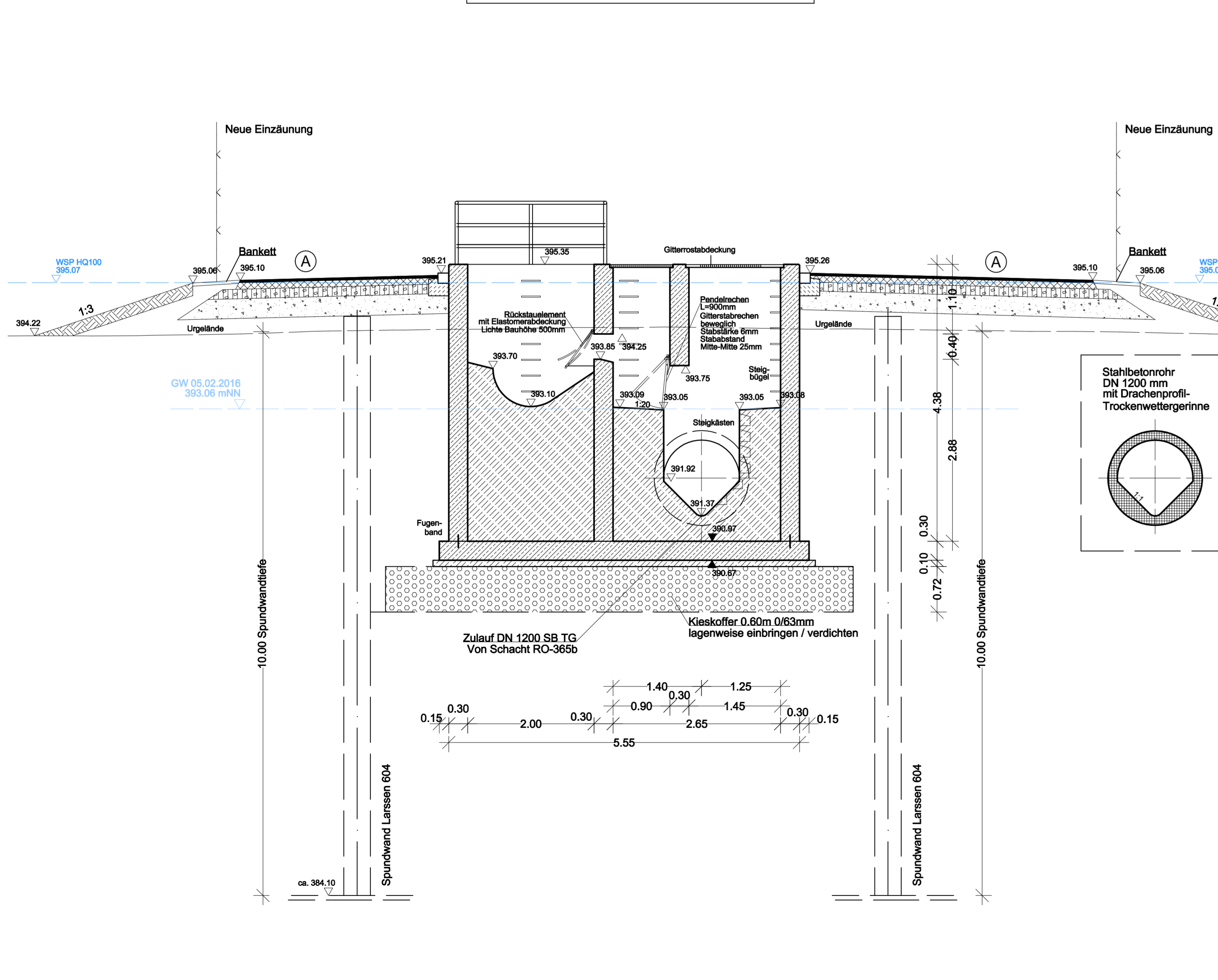
SCHNITT E-E
