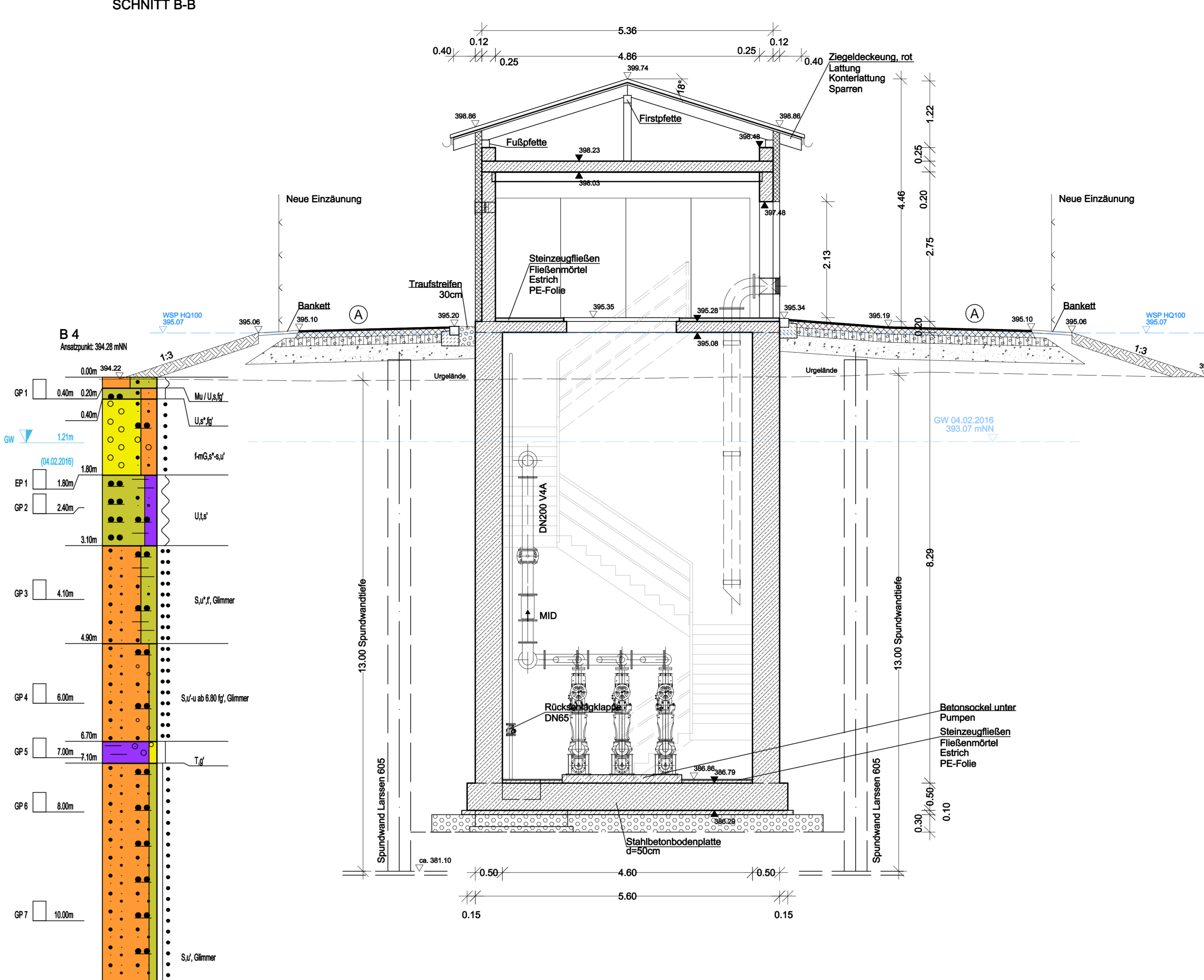
SCHNITT B-B
