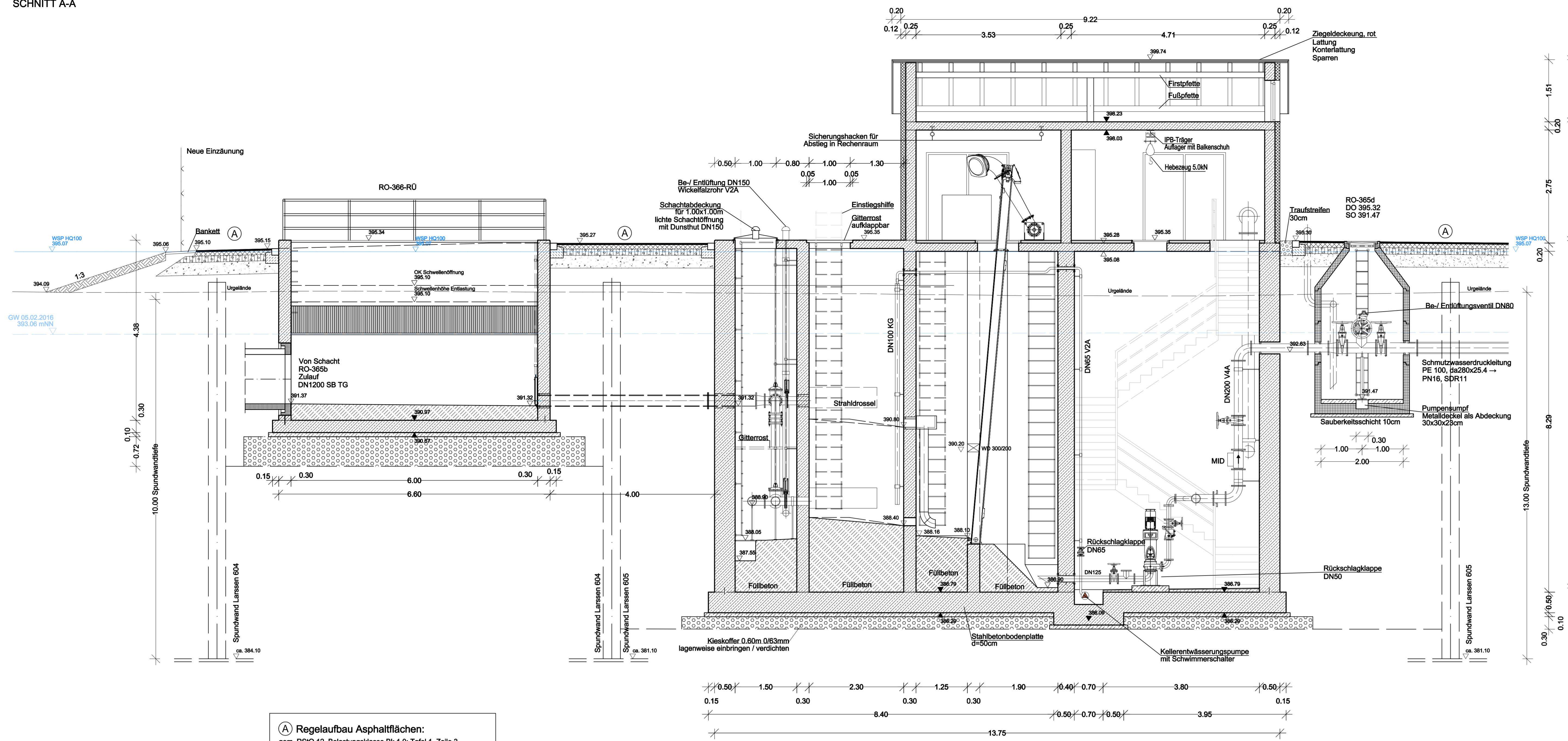
SCHNITT A-A
